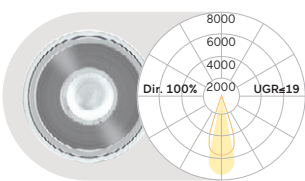
Contour Frame Lens 24°- 32°
